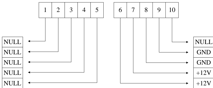
C330端子图：
