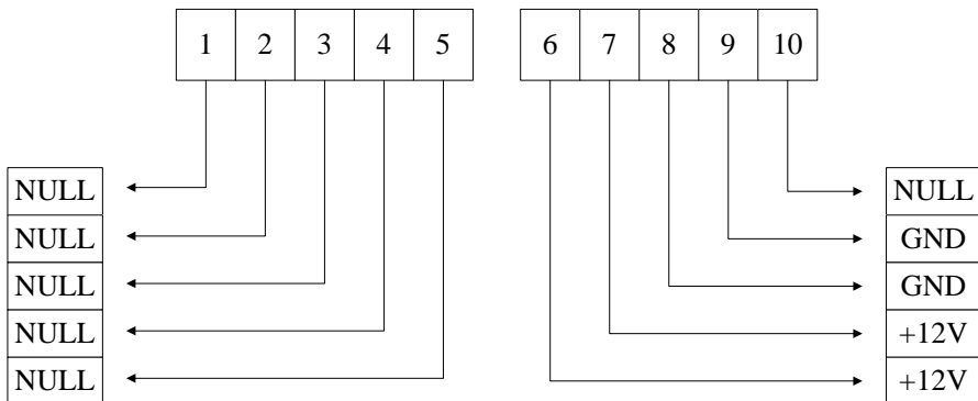
C330端子图:
